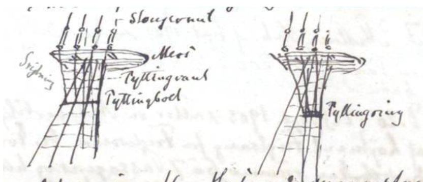
Tegning af kirkeskibets rigning
